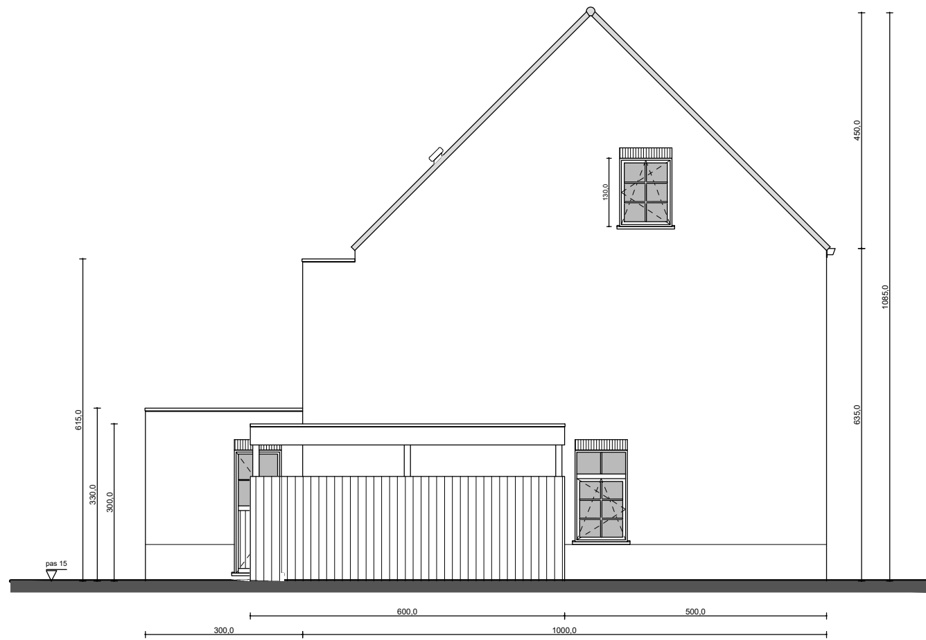
ZIJGEVEL LINKS
