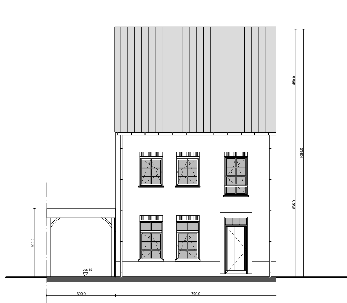
VOORGEVEL
