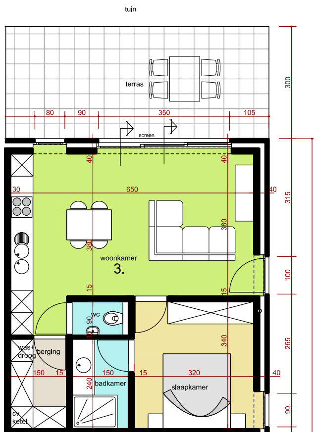
Grondplan
